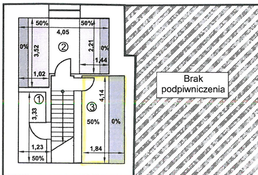
Szkic piwnic
